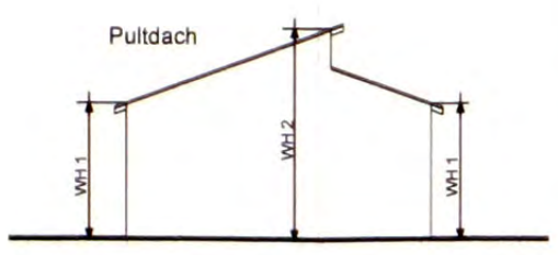
SCHEMASKIZZEN ZU WANDHÖHEN:
